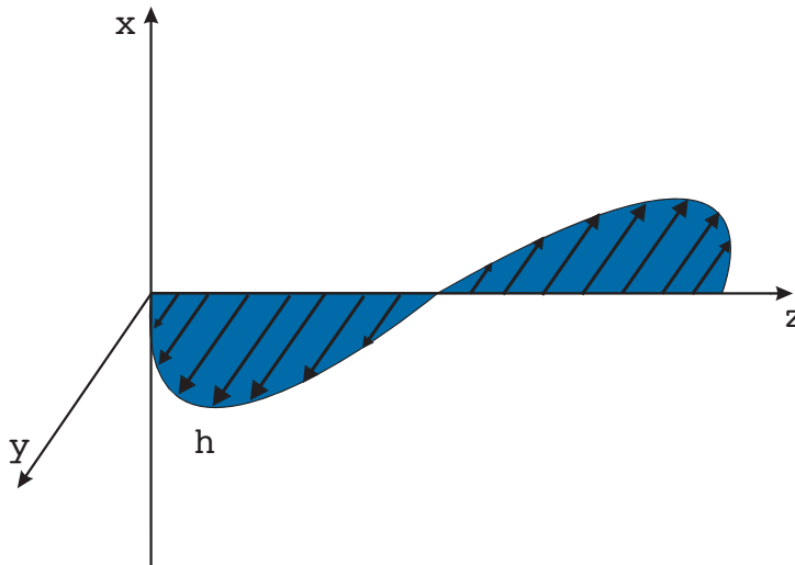
Abb. 3: Elektrisches Feld in Abstrahlrichtung z'
