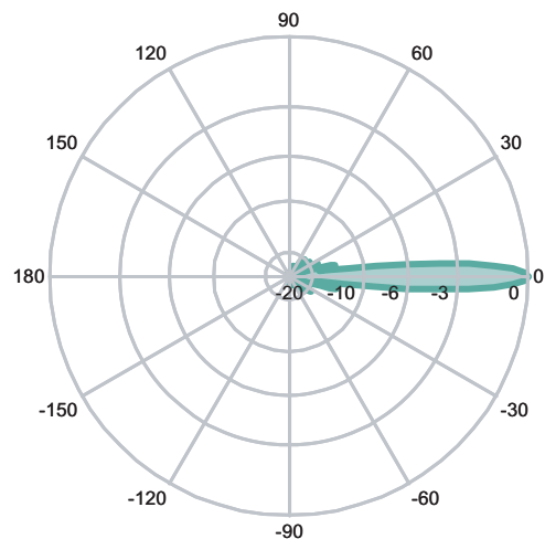
Anschluss: Vertikal / Polarisation: vertikal (5.470 MHz)
